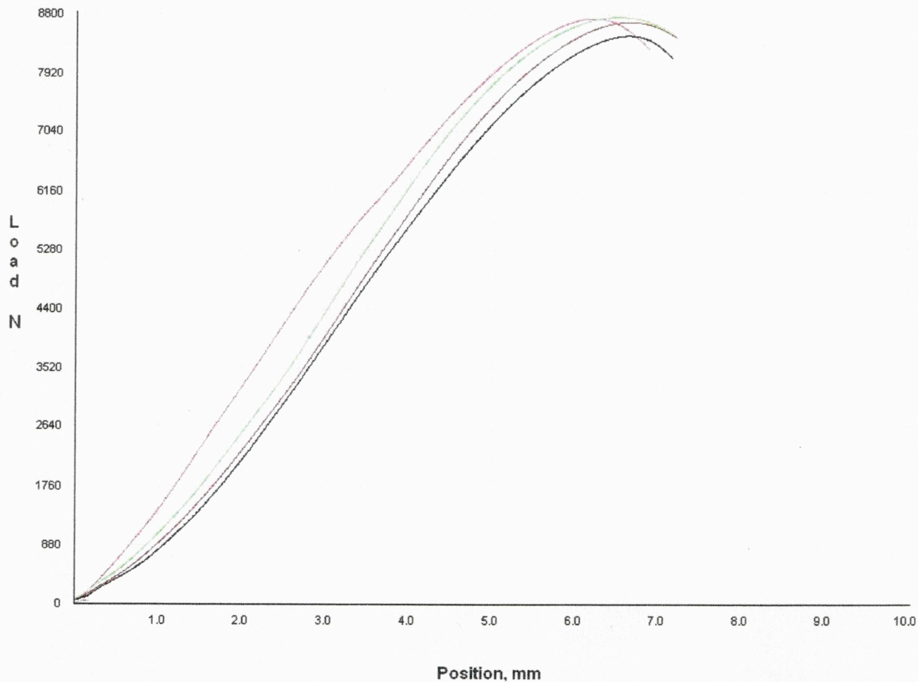
Fig. 2. Kraft/deformasjonsforløp ved belastning av 200 mm stag
